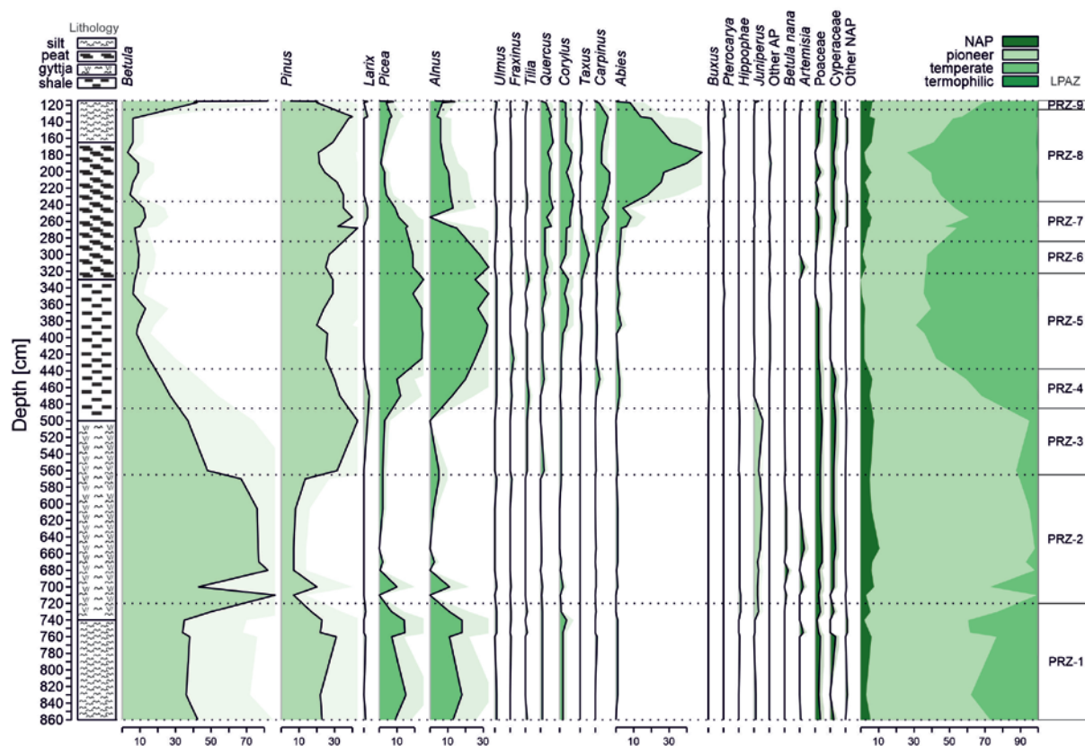
Text-fig. 10. Pollen diagram for Przytulín (H. Winter).
