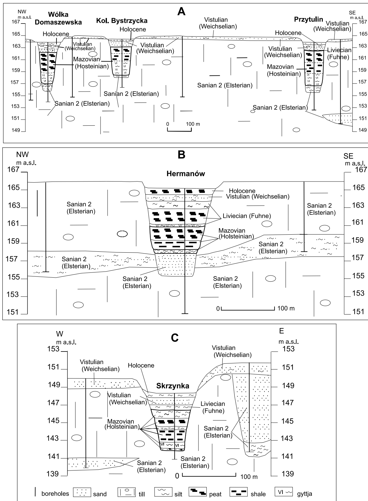
Text-fig. 5. Geological cross-section: A – Wólka Domaszewska-Przytulín, B – Hermanów, C – Skrzynka.
